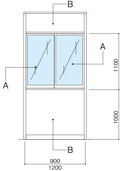
引き違いサッシ 平断面図 A-A
