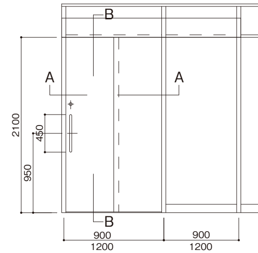
2連式ハンガードア 縦断面図
