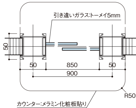
横断面図 A-A
