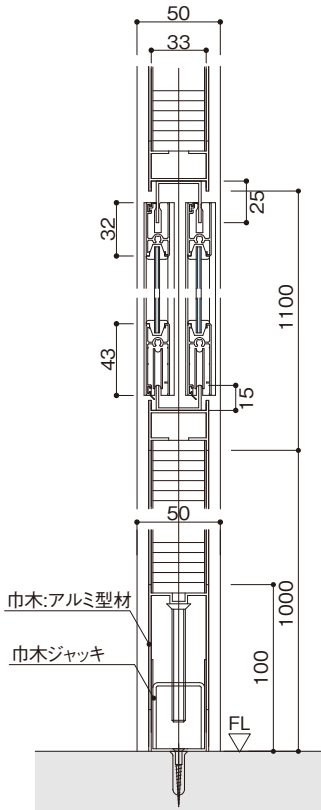
引き違いサッシ 縦断面図 B-B
