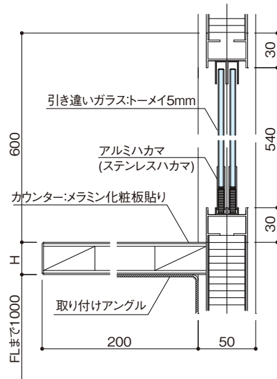
縦断面図 B-B
